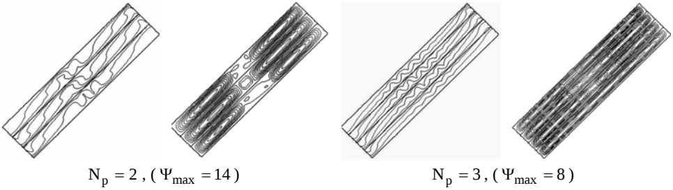
Fig. 3: Isothermes et lignes de courant: b = 0.08 m, \Delta T = 30 K et \varepsilon = 1
