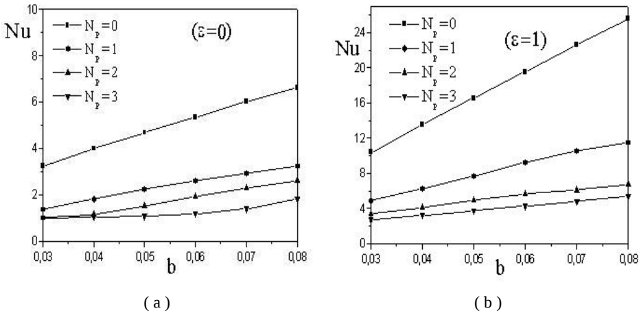
Fig. 4: Effet de la largeur de la cavité b , avec \Delta T = 30 K
