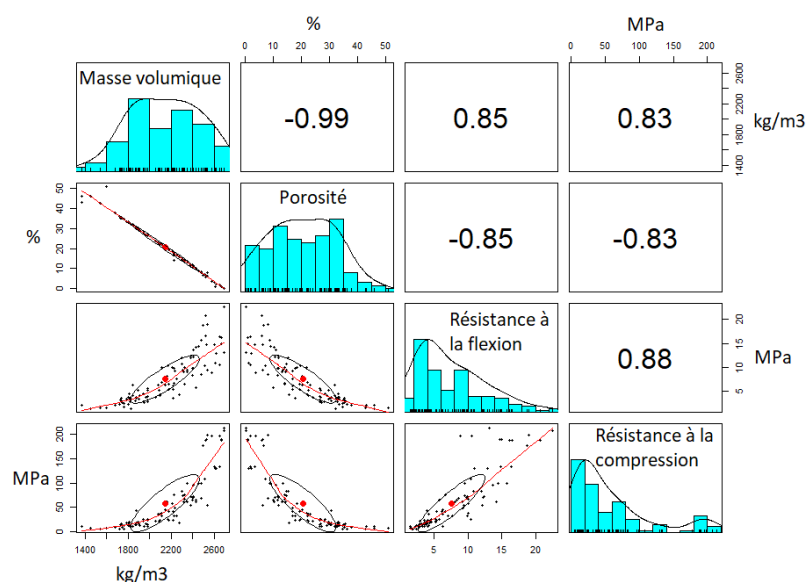
Figure 5 Corrélations des propriétés physiques des pierres calcaires
