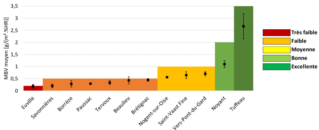
Figure 4 Capacité tampon hydrique (MBV) des pierres étudiées
