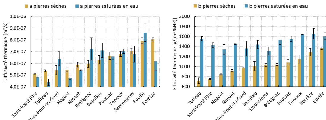
Figure 2 Diffusivité et effusivité thermique
