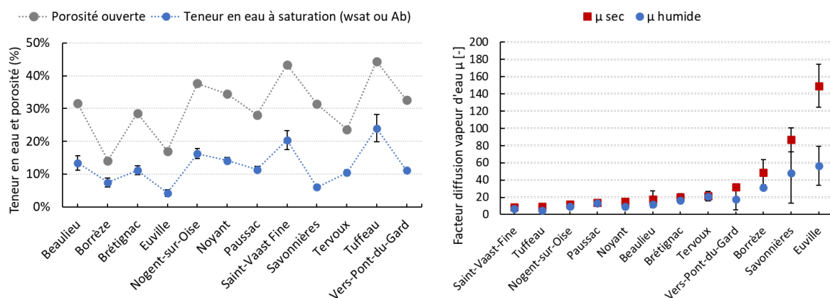
Figure 3 Porosité, absorption d'eau et facteurs de diffusion de la vapeur d'eau
