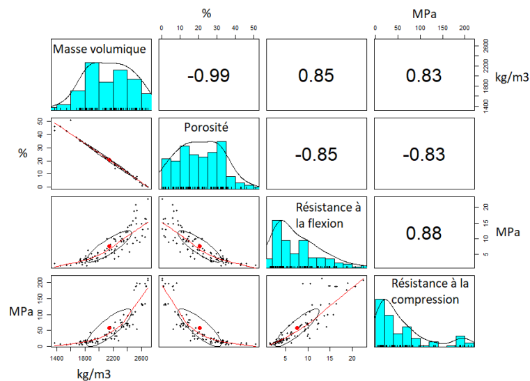
Figure 5 Corrélations des propriétés physiques des pierres calcaires
