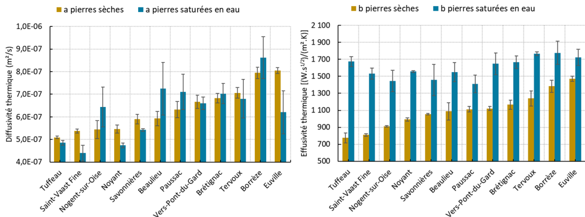
Figure 2 Diffusivité et effusivité thermique
