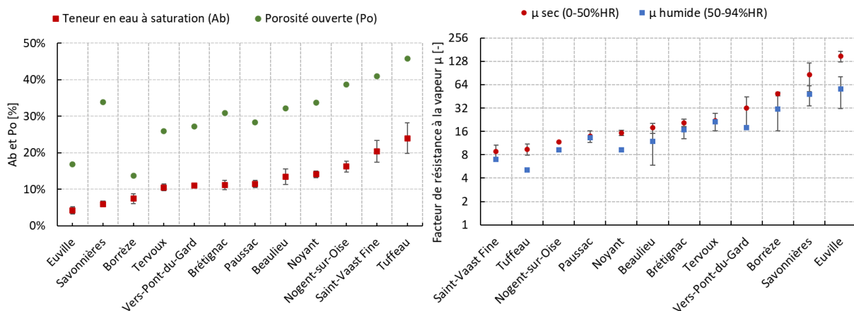
Figure 3 Porosité ouverte, teneur en eau à saturation et facteur de résistance à la vapeur d'eau
