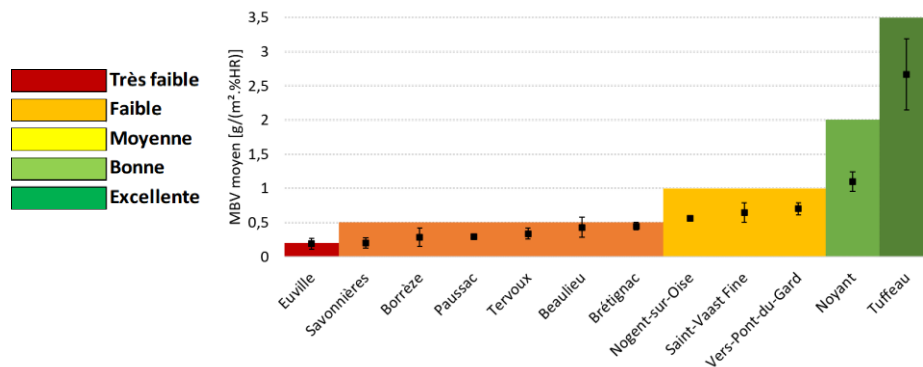
Figure 4 Capacité tampon hydrique (MBV) des pierres étudiées
