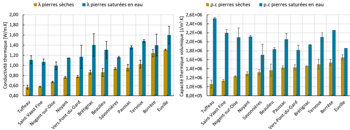
Figure 1 Conductivité et capacité thermique des pierres calcaires
